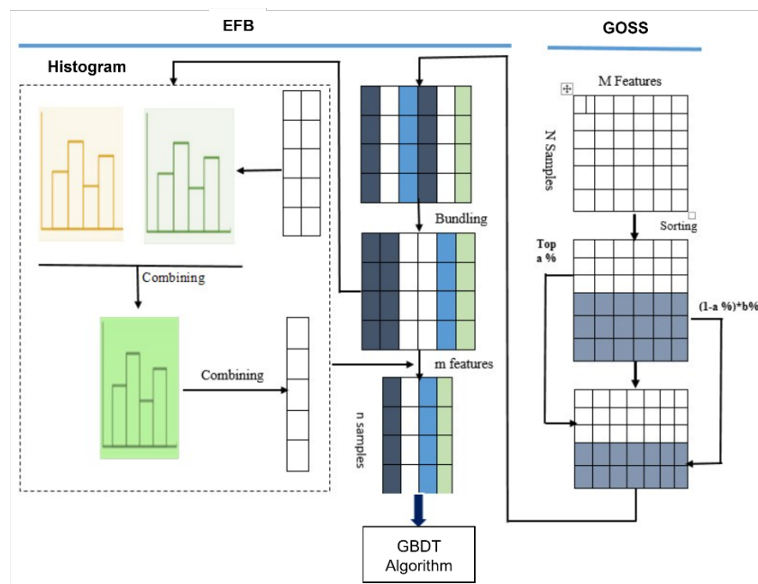
Gambar 2.4 Arsitektur GOSS dan EFB
