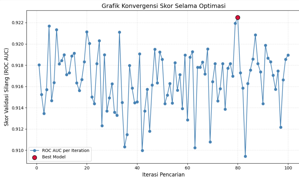
Gambar 4.24 Grafik Konvergensi Skor Selama Optimasi
