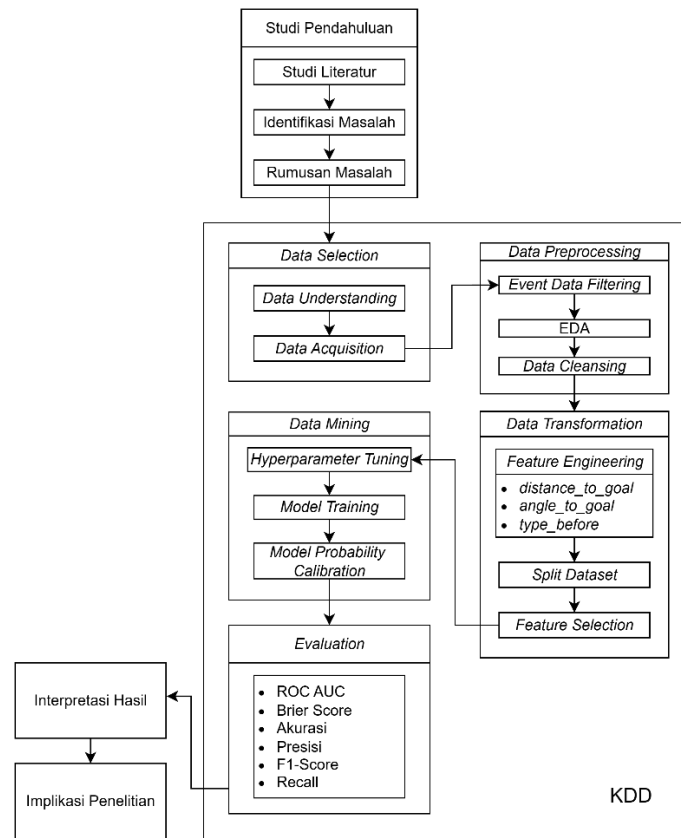
Gambar 3.1 Tahapan Penelitian
