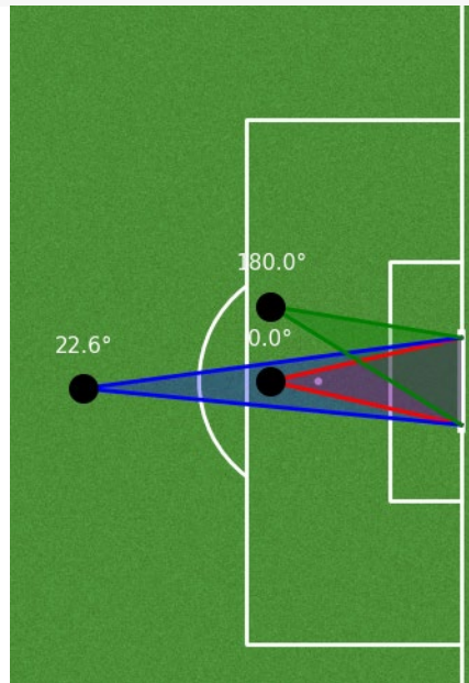
Gambar 4.20 Visualisasi angle_to_goal
